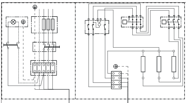
Anschlussplan für 7,5 kW Ofen (bei 6 kW 3 Rohrheizkörper à 2000 W)
