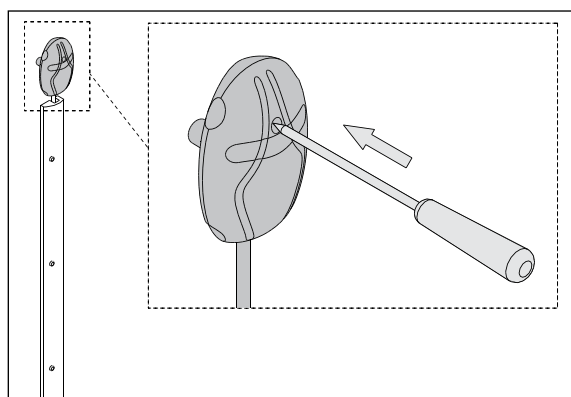
Figure 13. Reset button for overheat protector Abbildung 13. Rücksetzknopf des Überhitzungsschutzes
