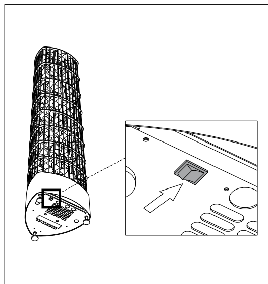
Figure 8. Main switch Abbildung 8. Hauptschalter
