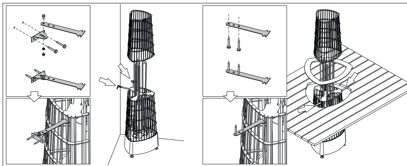
Figure 12. Fixing the heater with fixing kits Abbildung 12. Anbringen des Ofens mit Befestigungssätzen
