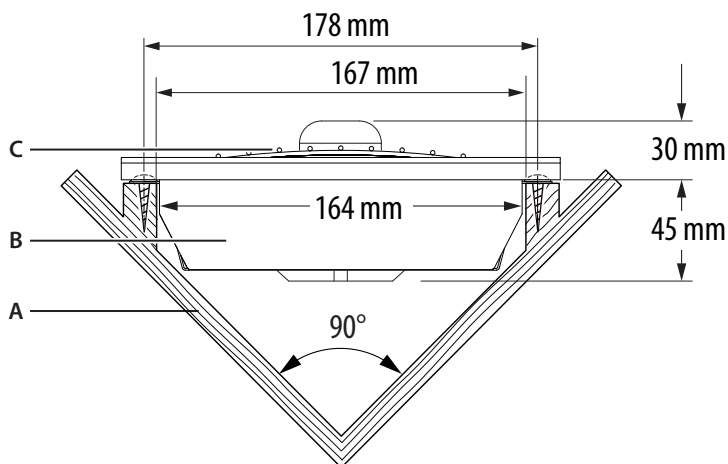
Einbau in die Kabinenecke
