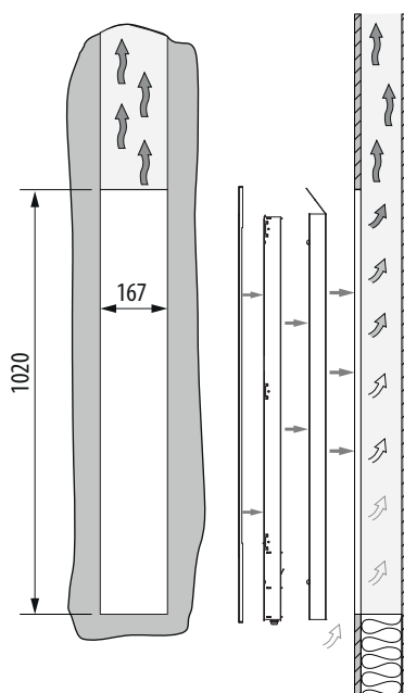
Einbauöffnung und Wandkonstruktion
