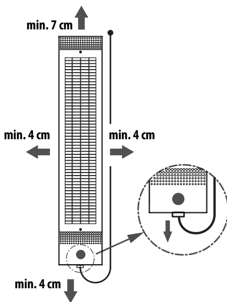
Vitae Protect+ - Mindestabstände zu brennbaren Materialien. Kabelanschluss nach unten.
