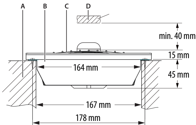
Einbau in die Kabinenwand
