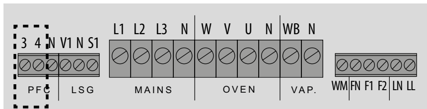
Anschluss Potentialfreier Kontakt
