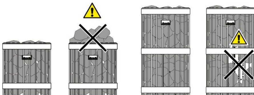
Rysunek 7. Sposób układania kamieni w saunie
