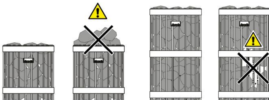
Obrázek 7 Umístění saunových kamenů
